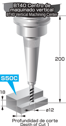
Portaherramienta Hidráulico Delgado Slim Hydro Chuck
